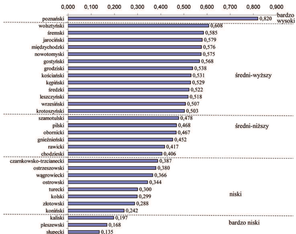
Rysunek 1. Uporządkowanie liniowe powiatów województwa wielkopolskiego według poziomu rozwoju społeczno-gospodarczego oraz ich klasyfikacja typologiczna (metoda TOPSIS)
